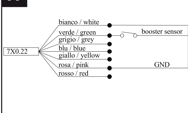
Alimentazione (fig.18)
