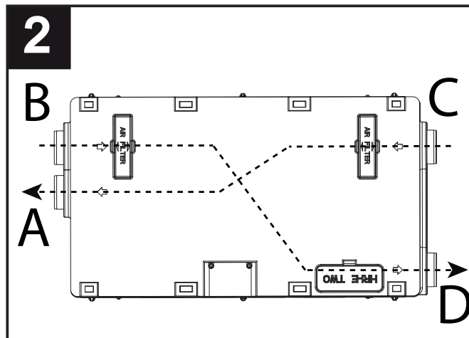
Popis otvorů průchodu vzduchu (obr.2)
