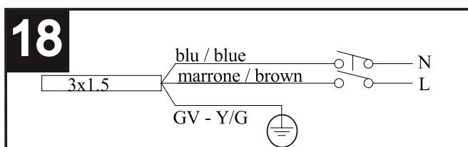
Alimentation (fig.18)
