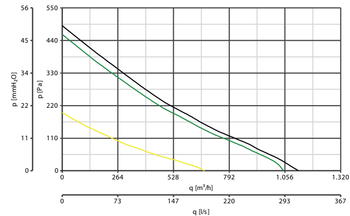
CA 200 ES CODE 16175 - MAX SPEED
