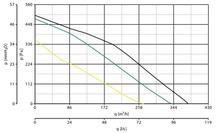
CA 125 ES CODE 16171 - MAX SPEED
