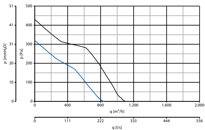
LINEO 200 Q V0
