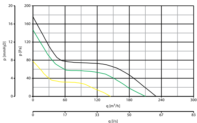
LINEO 100 ES CODE 17031 - MAX SPEED
