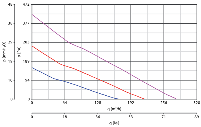
CA 125 ES CODE 16171 - MIN SPEED
