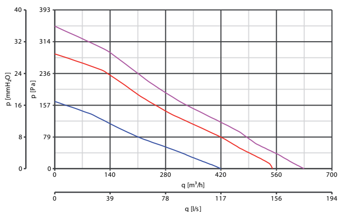
CA 160 ES CODE 16174 - MIN SPEED
