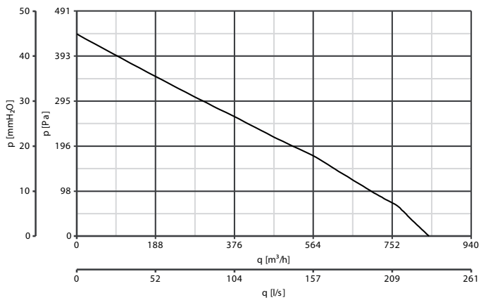
CA 315 V0 E CODE 16041
