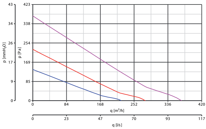
CA 150 Q ES CODE 16172 - MIN SPEED
