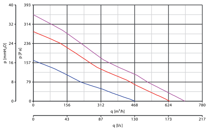
CA 200 ES CODE 16175 - MIN SPEED
