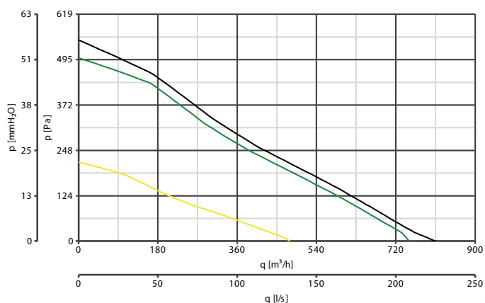
CA 160 ES CODE 16174 - MAX SPEED
