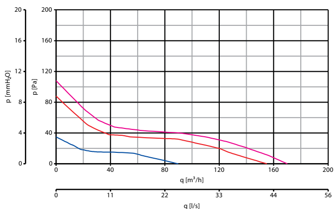
LINEO 100 ES CODE 17031 - MIN SPEED
