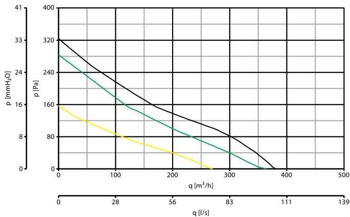
LINEO 125 ES CODE 17032 - MAX SPEED
